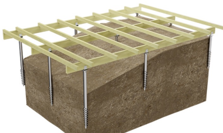
Etape 3 : Double lambourdage
