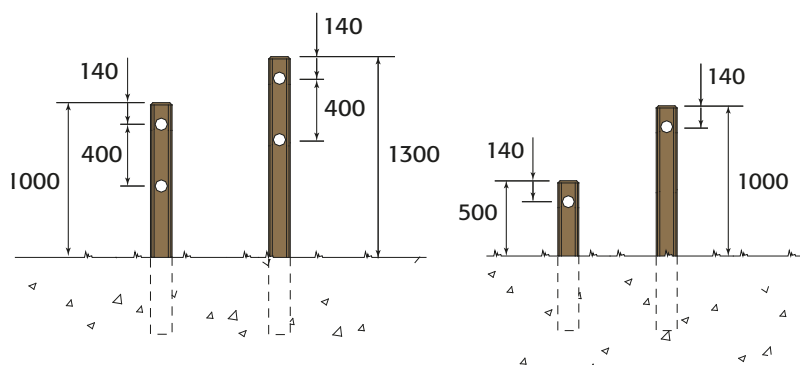
Clôture pré-percée
