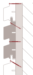
Vibrato XL
